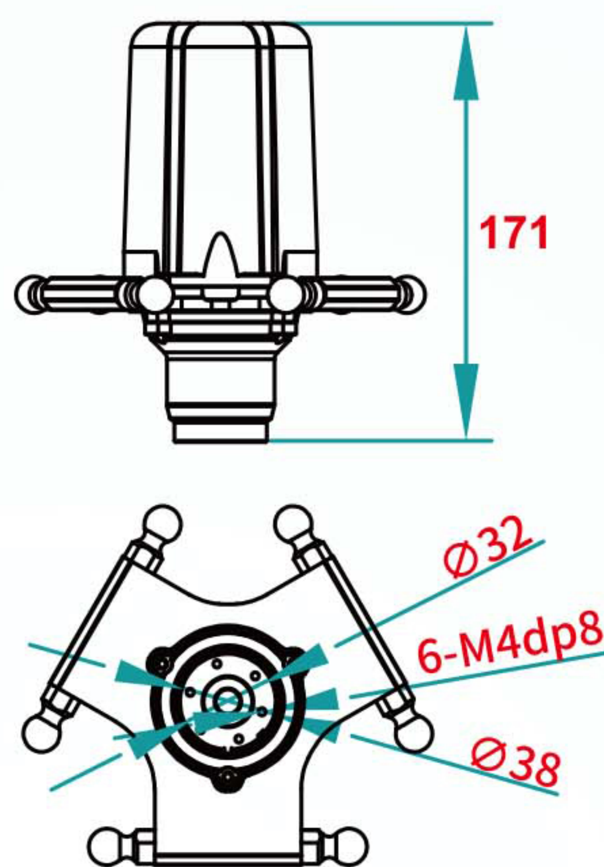
末端法兰 End Flange
